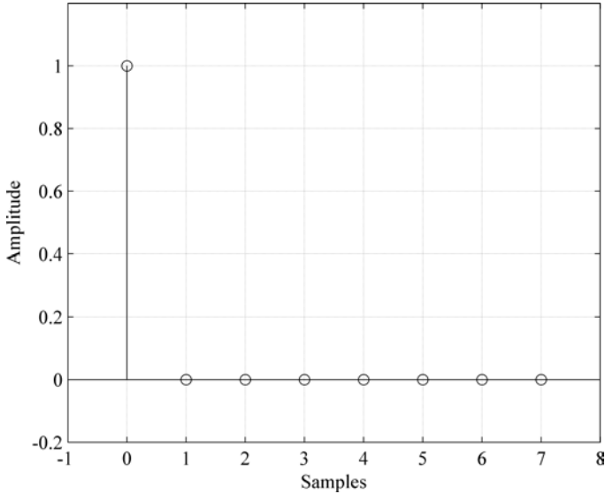
Fig. 4.1. Impulse signal.
