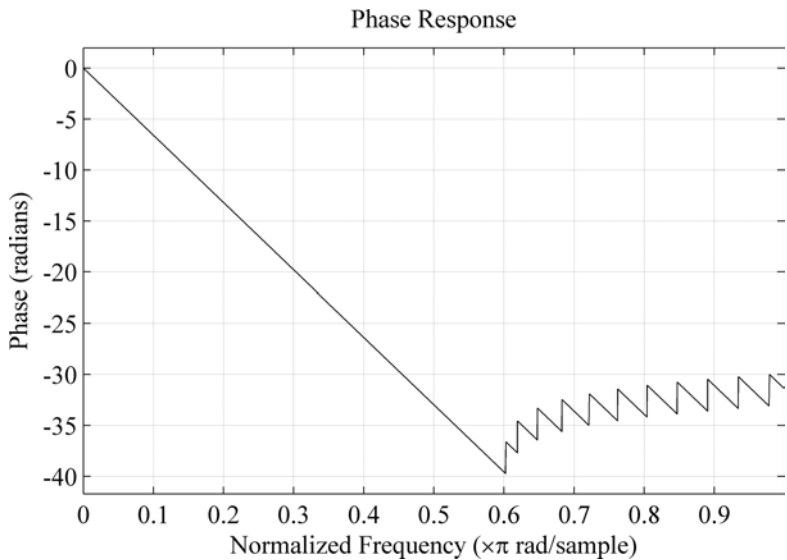
Fig. 2.7. LPF FIR phase response.
